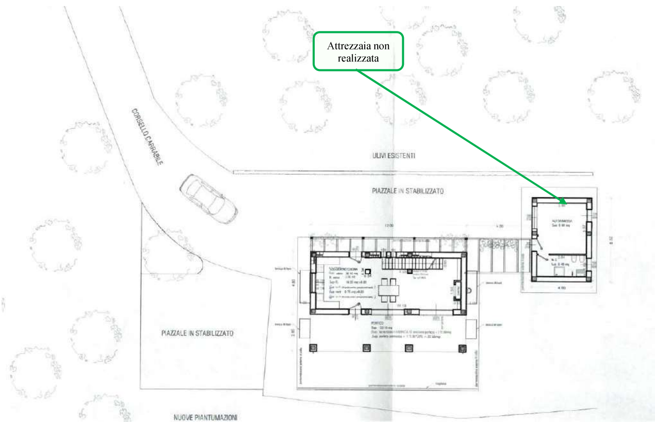
planimetria e collocazione del fabbricato
