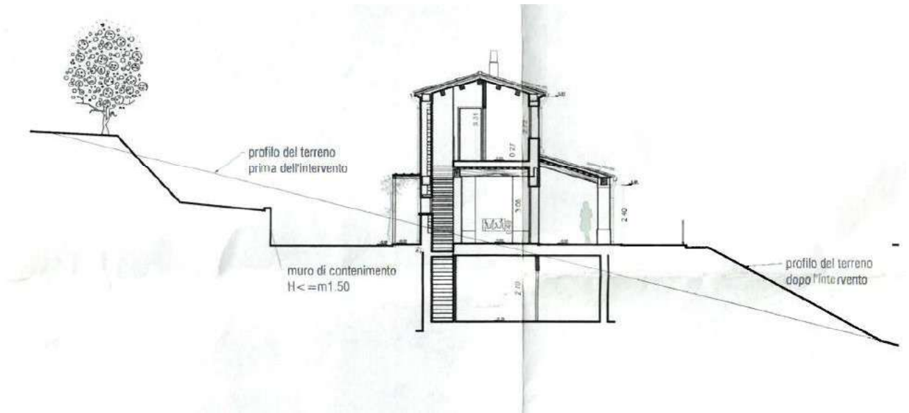
sezione del fabbricato
