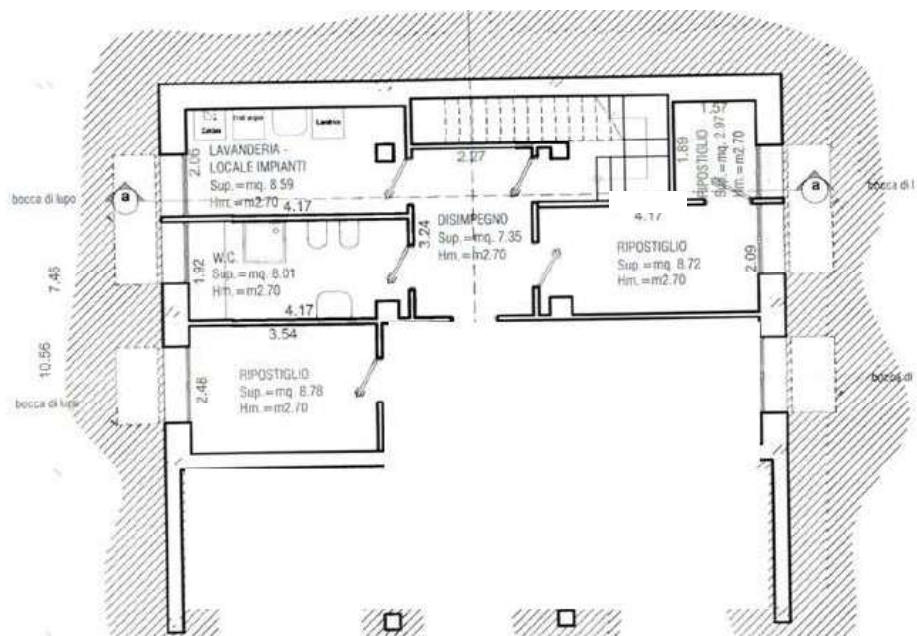
Edificio - pianta piano interrato - stato dei luoghi
